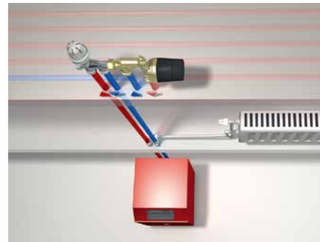
散热器安装示意
